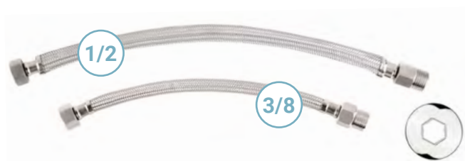
Ligação flexível Fluid - 1/2 trançado inox - com espelho ½ BSP [IxE]
